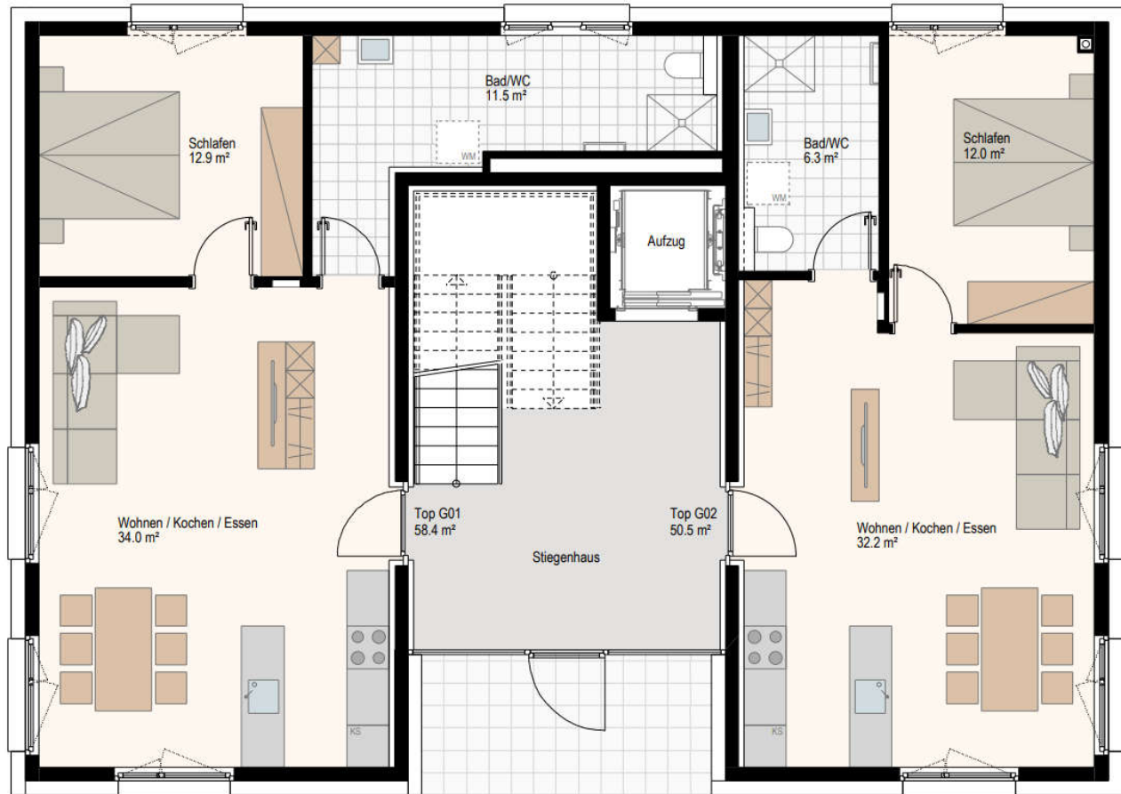
Haus C / Erdgeschoss
