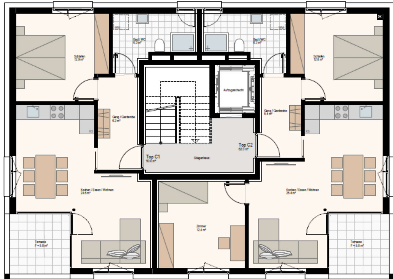
Haus C / 1.Obergeschoss
