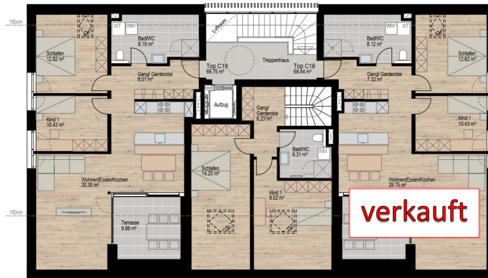
Variante 3-Zi-Wohnung
