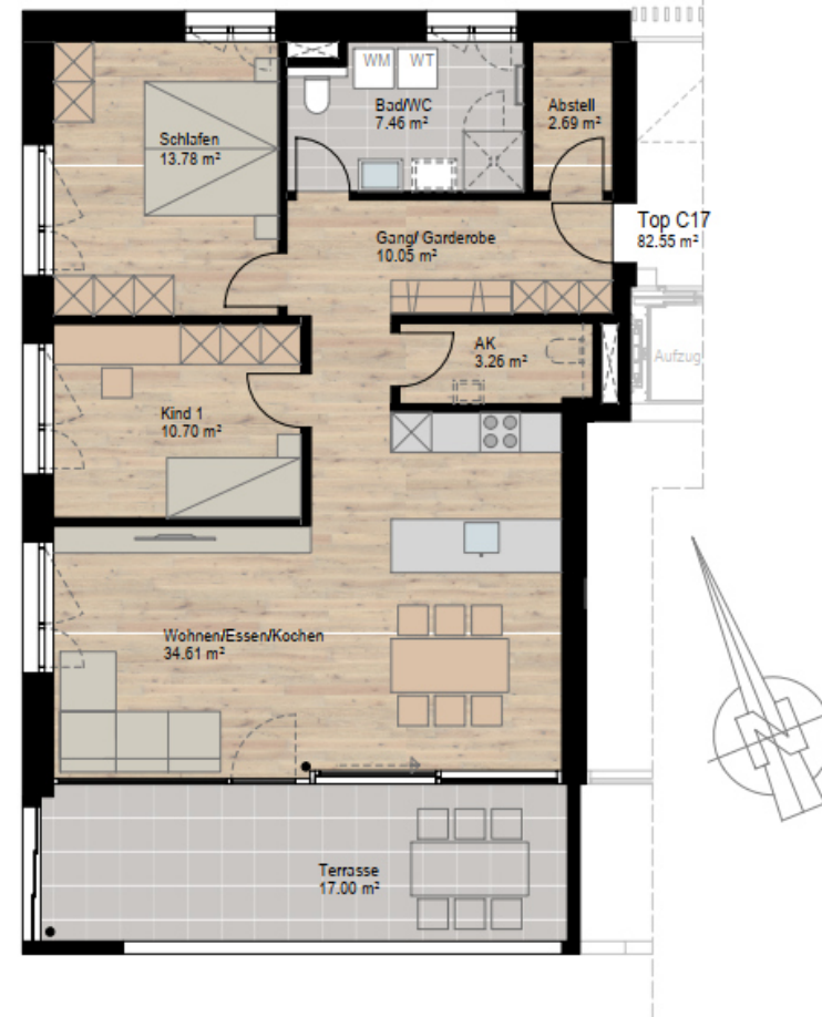
Variante 3-Zi-Wohnung
